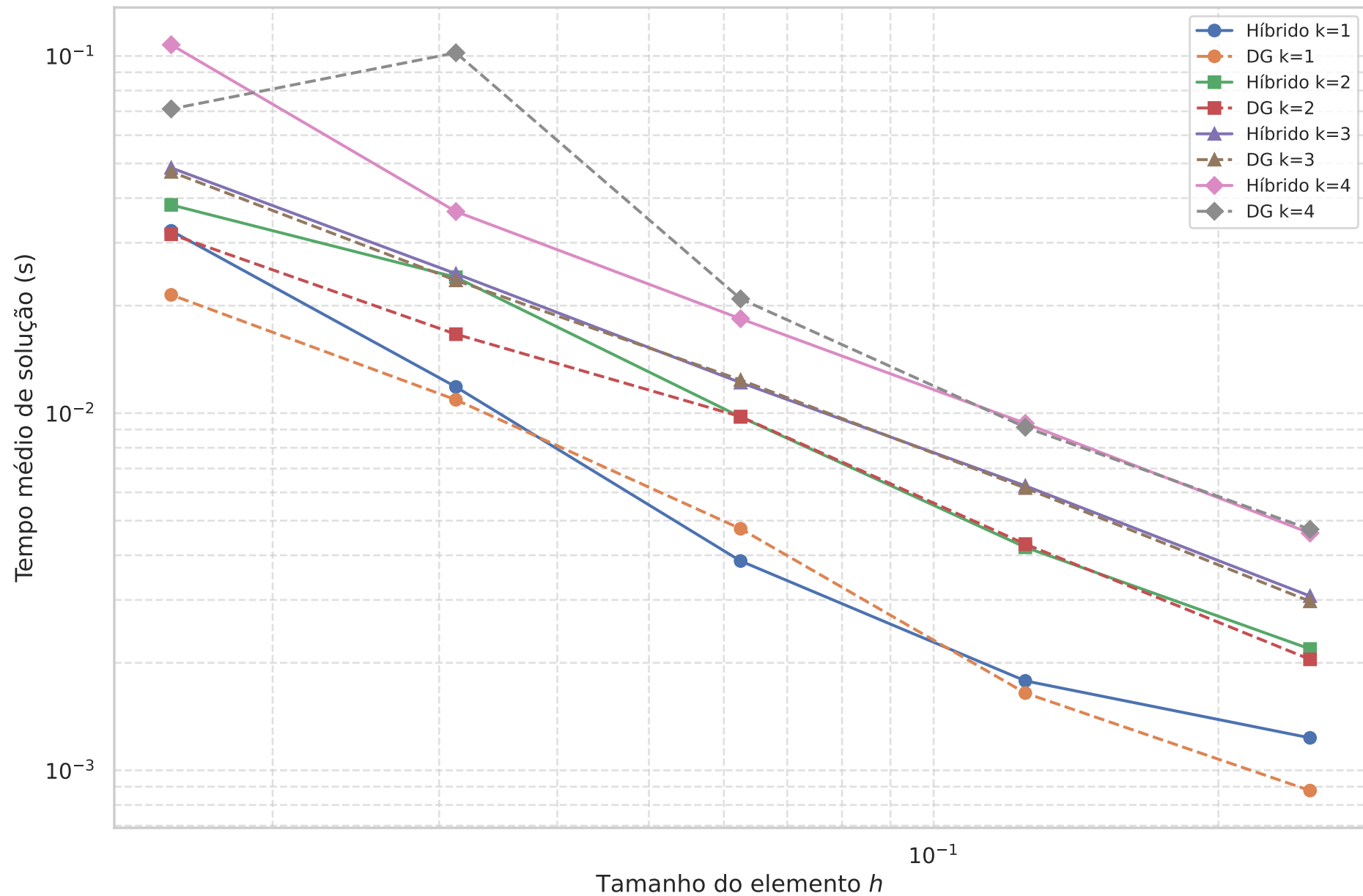
Custo computacional - Híbrido vs DG, \alpha = 0
