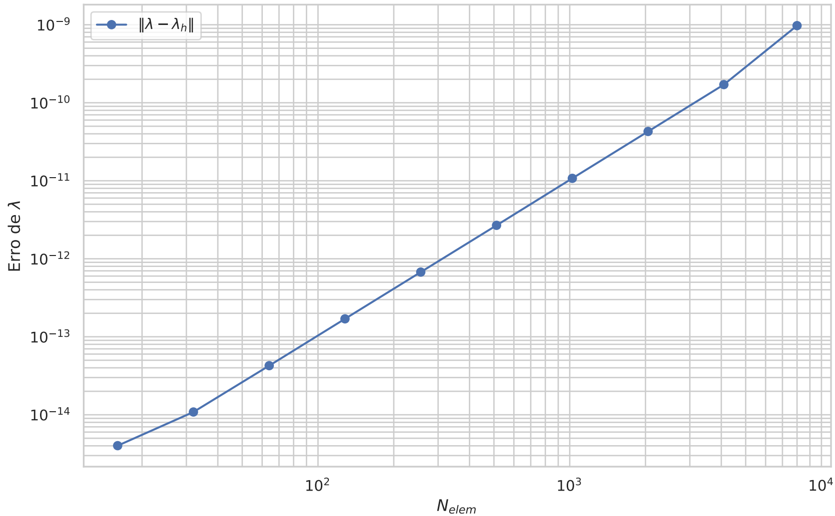
Item (e): erro de \lambda_h em função de N_{elem}
