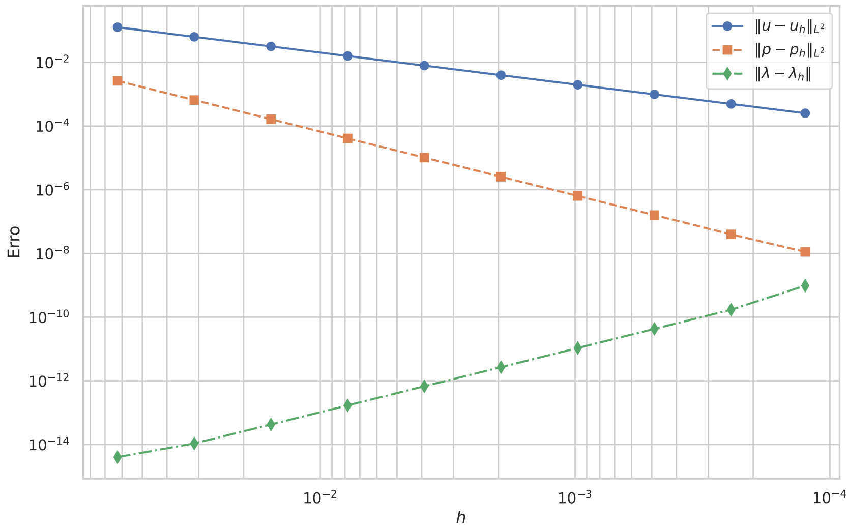
Item (e): erros de u_h , p_h e \lambda_h
