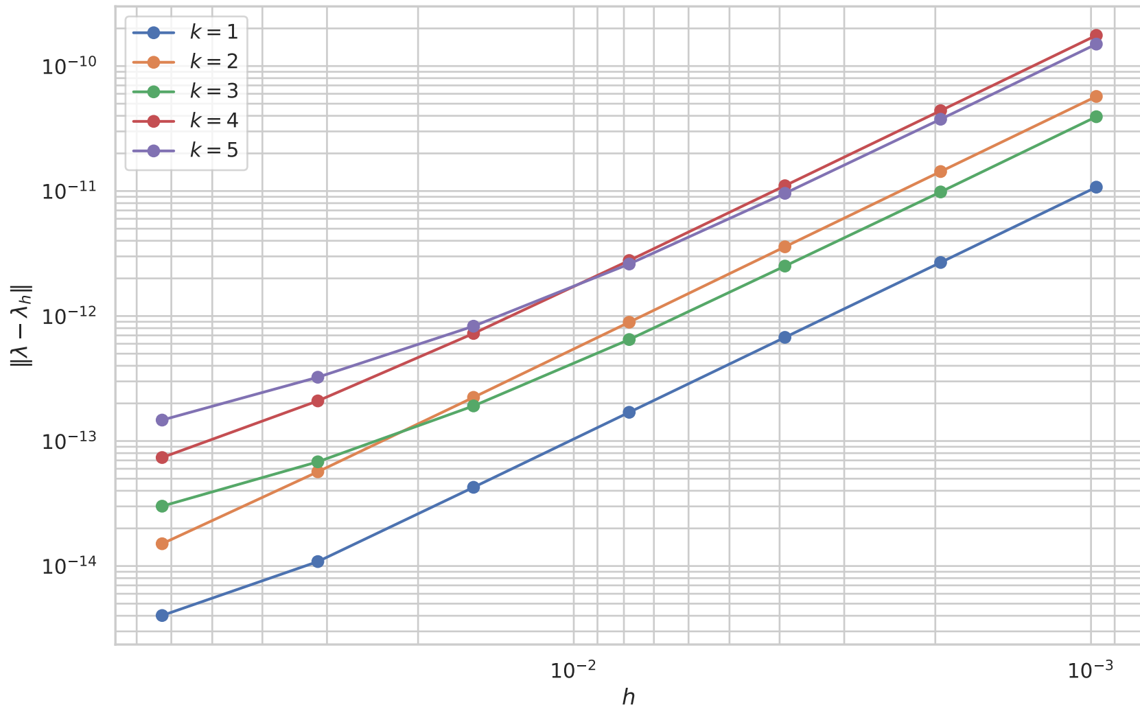
Item (f): erro de \lambda_h para k = 1, 2, 3, 4, 5
