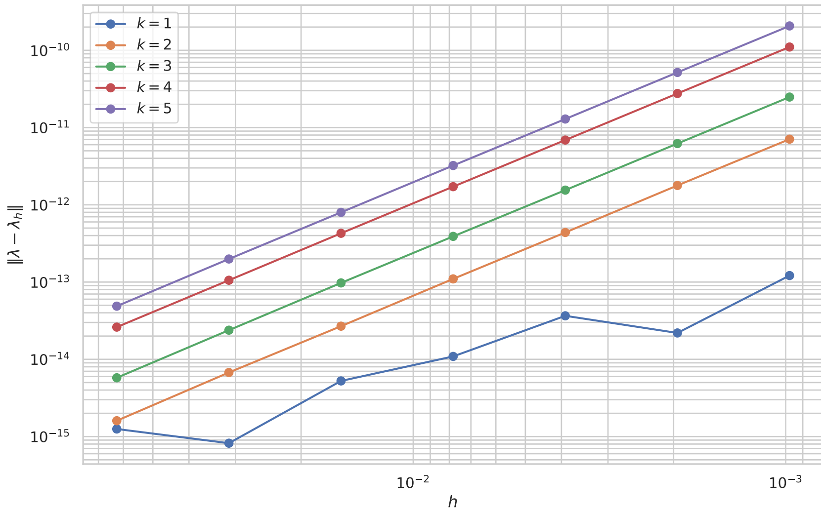
Item (g): erro de \lambda_h com \delta_1 = -1/2 e \beta = 0
