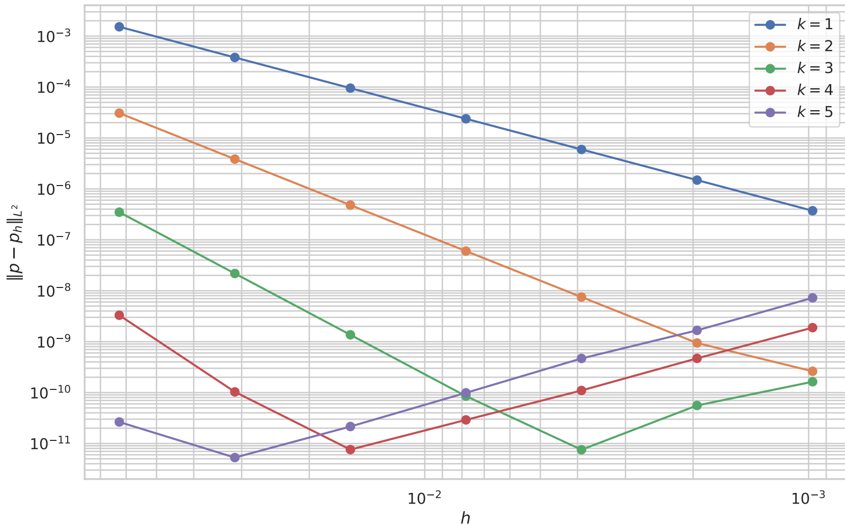
Item (i): erro de p_h usando \lambda_h aproximado por Poisson
