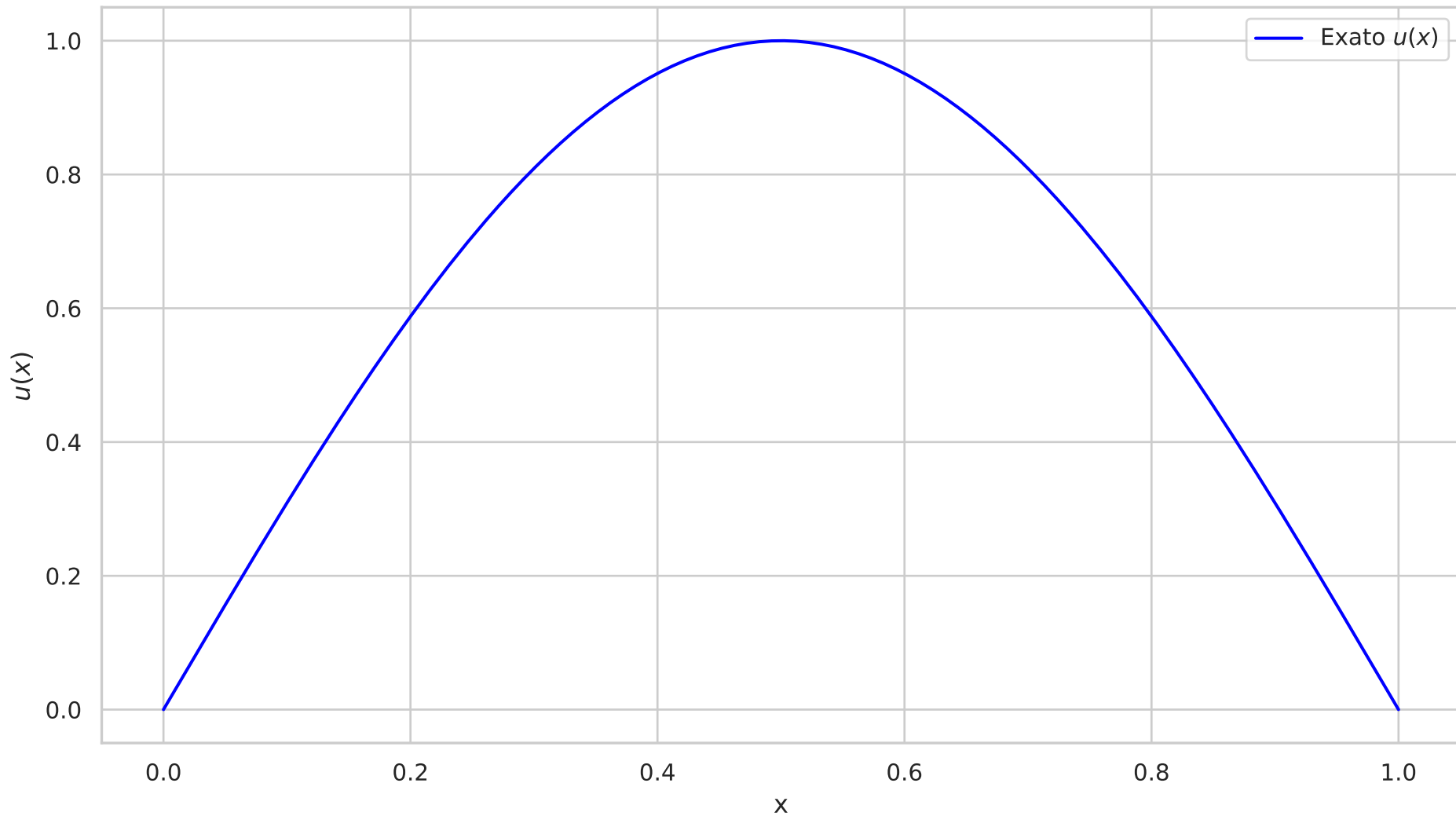
Solução exata u(x) = \sin(\pi x)
