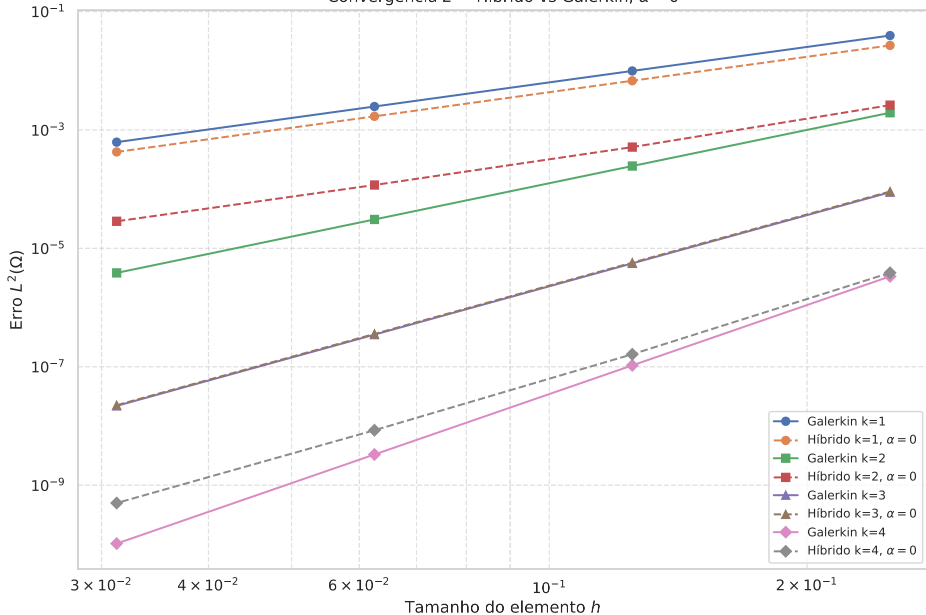
Convergência L^2 - Híbrido vs Galerkin, \alpha = 0
