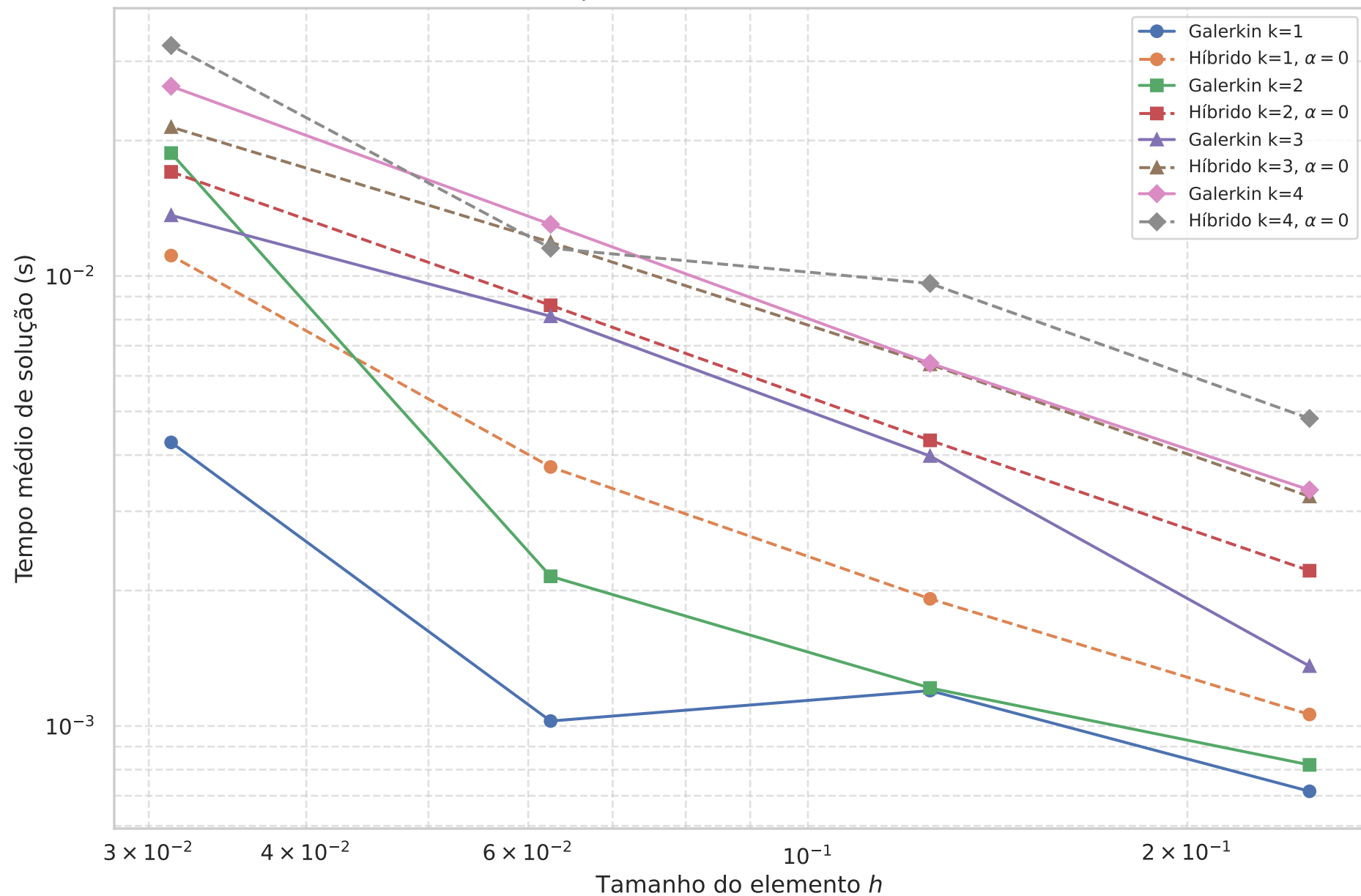
Custo computacional - Híbrido vs Galerkin, \alpha = 0
