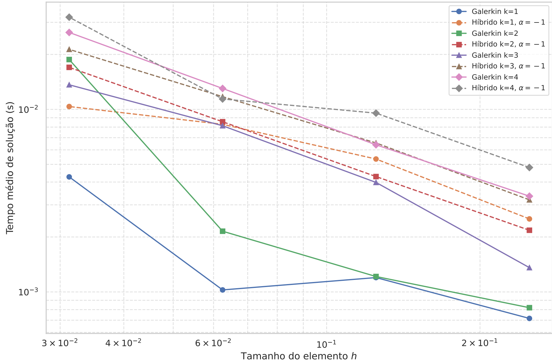
Custo computacional - Híbrido vs Galerkin, \alpha = -1
