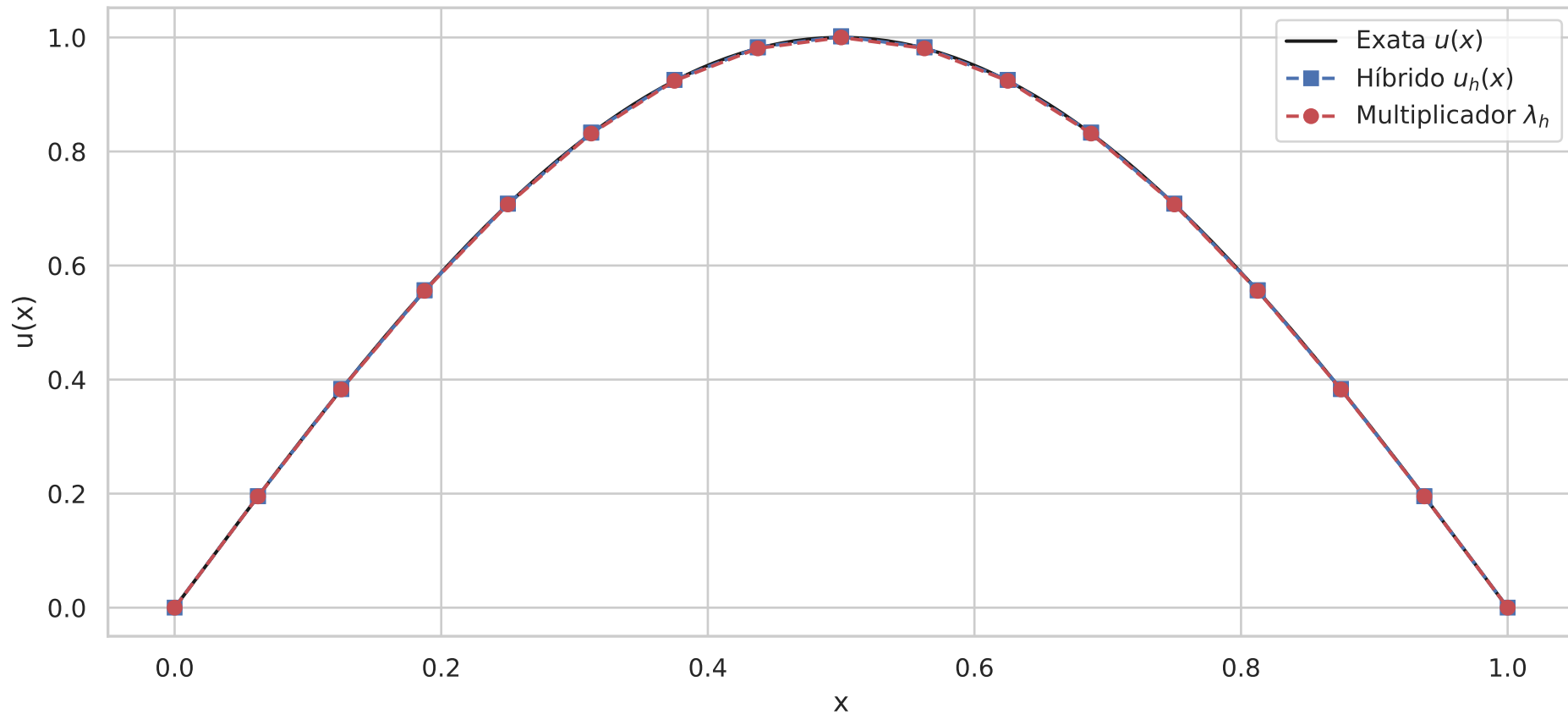
Método híbrido: N = 16 , k = 1 , \alpha = -1 , \beta = 1.60e + 02
