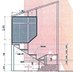
MALLA Y REFUERZOS EN GRADAS
