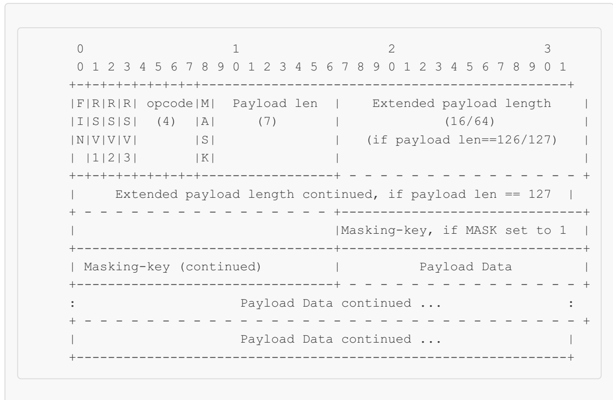
Diagrama de una trama de WebSocket, adaptado de RFC 6455.
