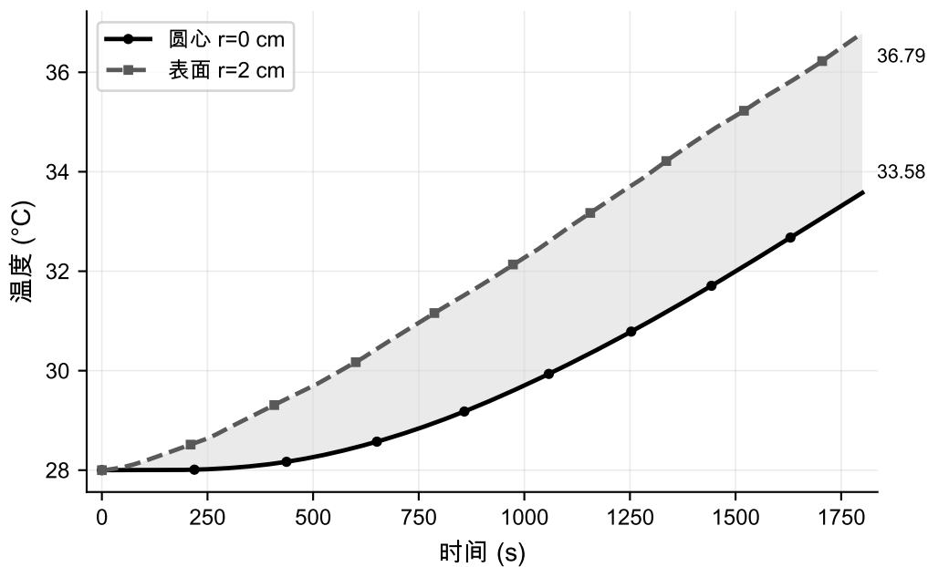
圆心与表面温度
