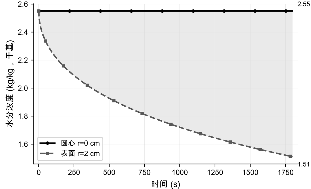
圆心与表面水分浓度
