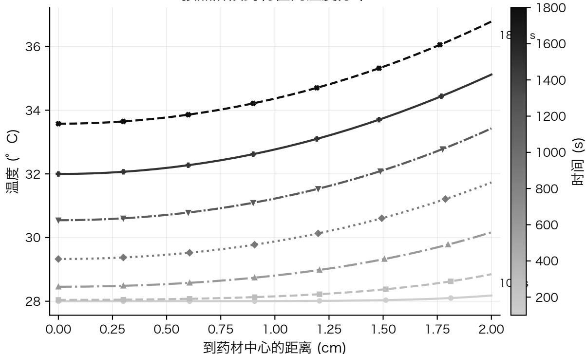
预热阶段药材径向温度分布
