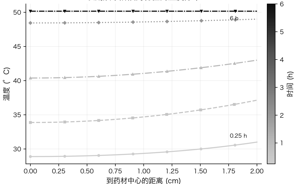
长期烘干阶段药材径向温度分布
