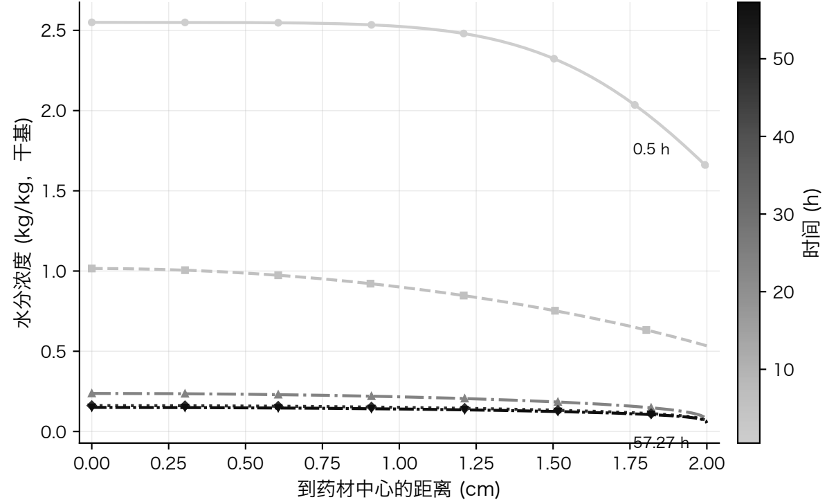
圆心与表面水分浓度
