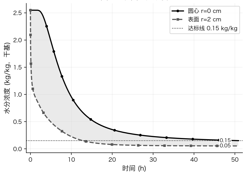
圆心与表面水分浓度
