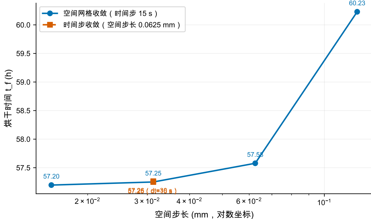
问题3：烘干时间对网格与时间步的收敛趋势
