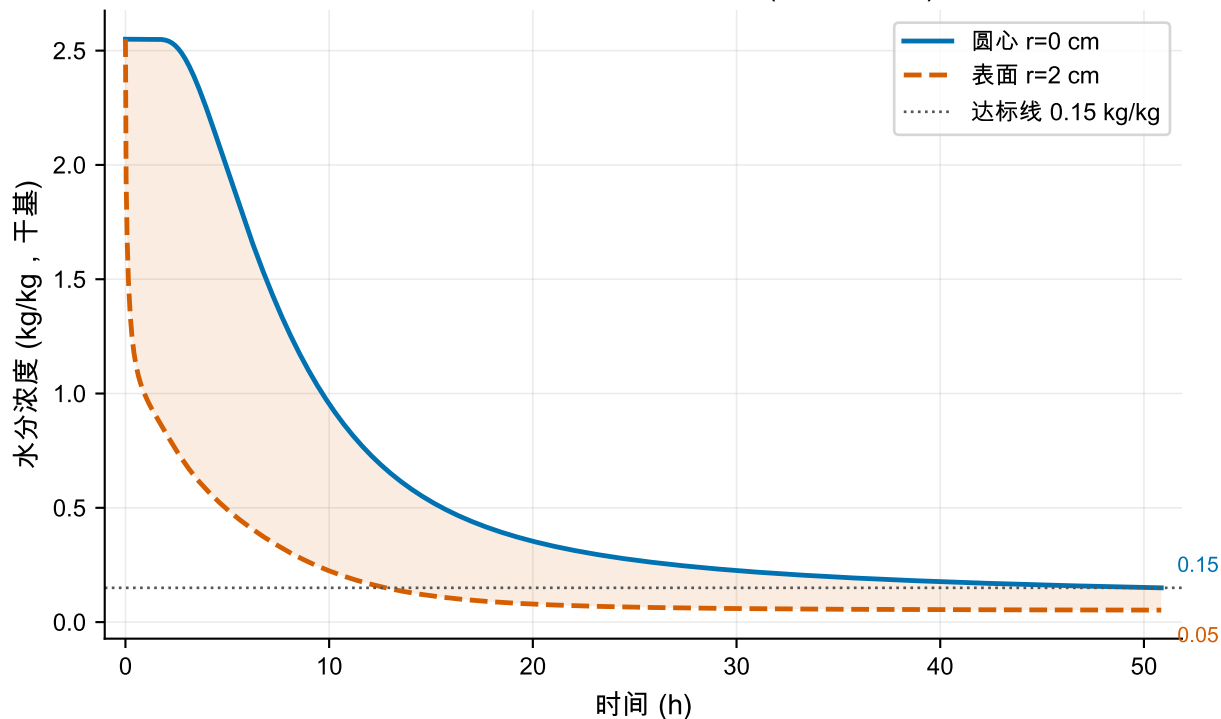
圆心与表面含水率随时间变化 ( 收缩条件 )
