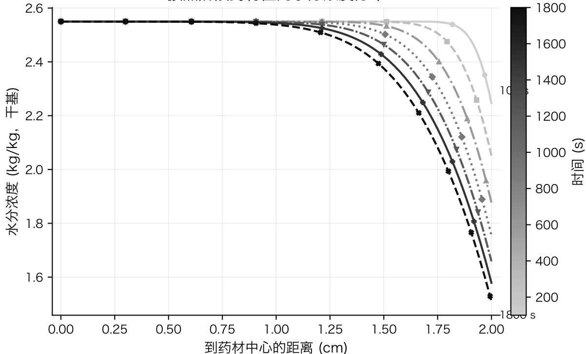
预热阶段药材径向水分浓度分布
