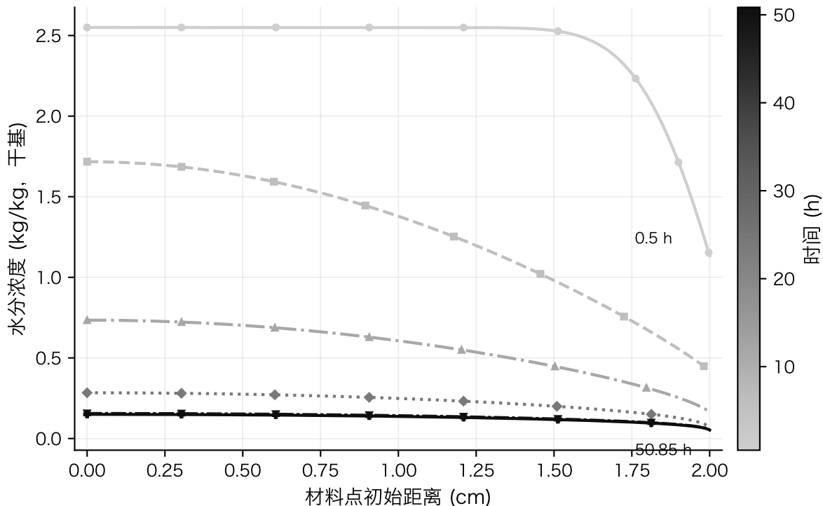
收缩条件下药材内部水分浓度分布（材料坐标）
