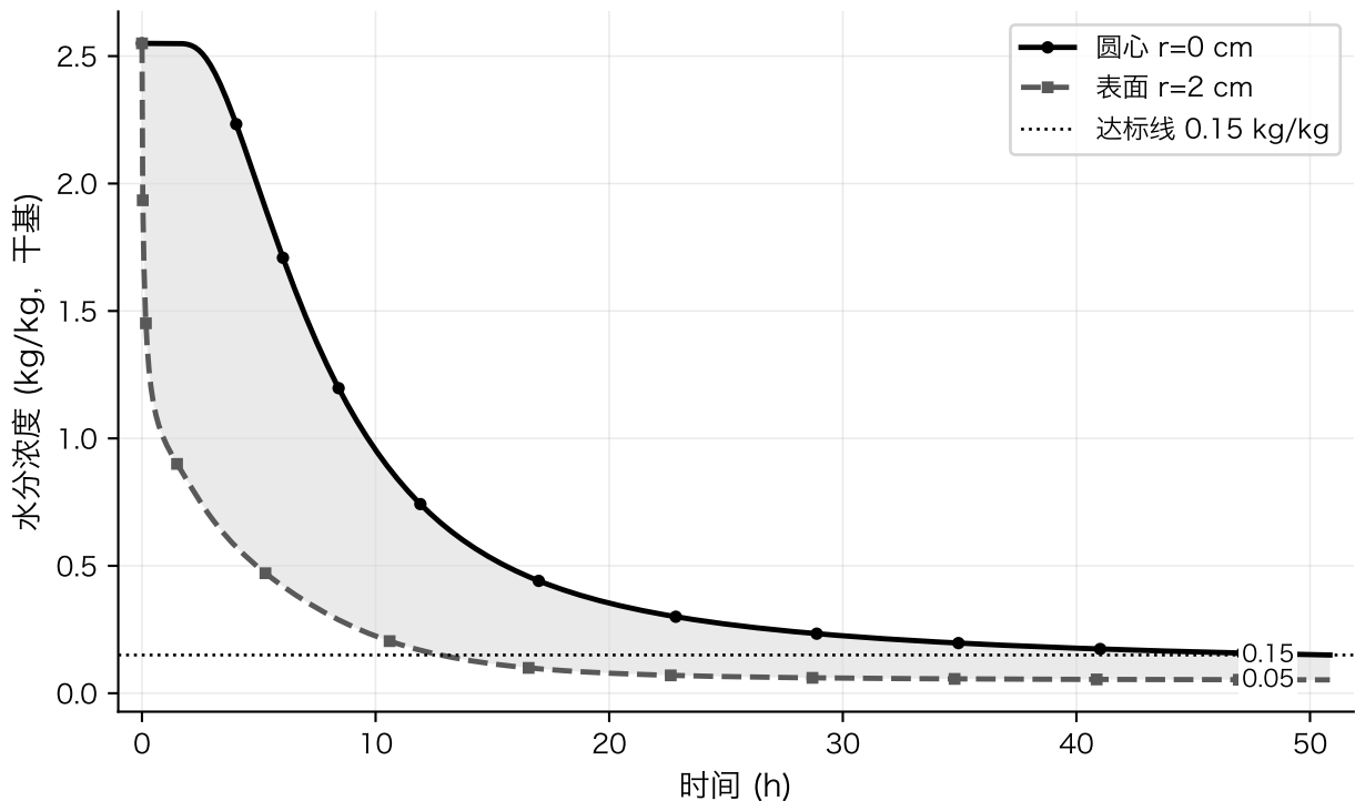
圆心与表面水分浓度随时间变化（收缩条件）
