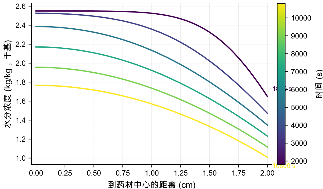
径向水分浓度分布
