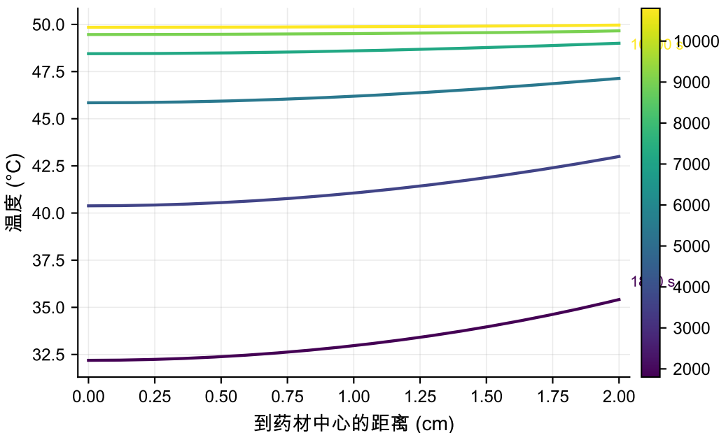
径向温度分布
