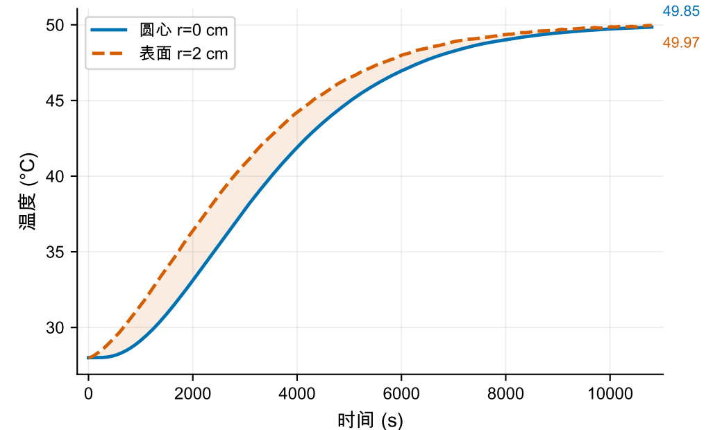
圆心与表面温度
