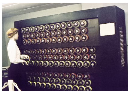
Une « bombe » de décryptage, Bletchley Park.
