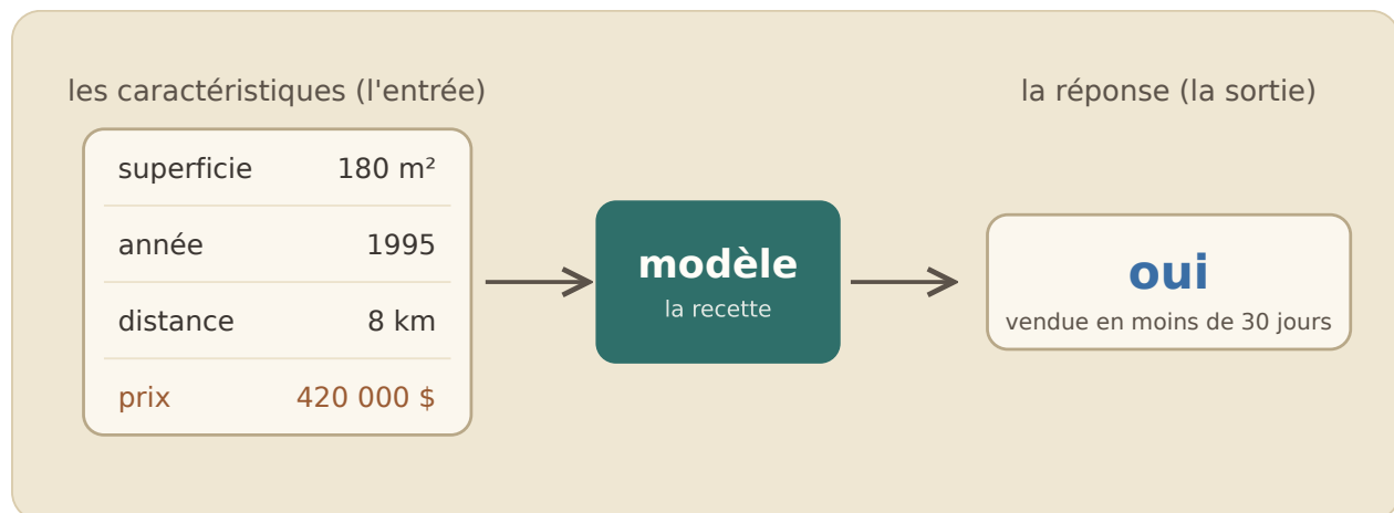
Figure 48: Le modèle de classification : les caractéristiques entrent, le prix compris ; une catégorie sort.
