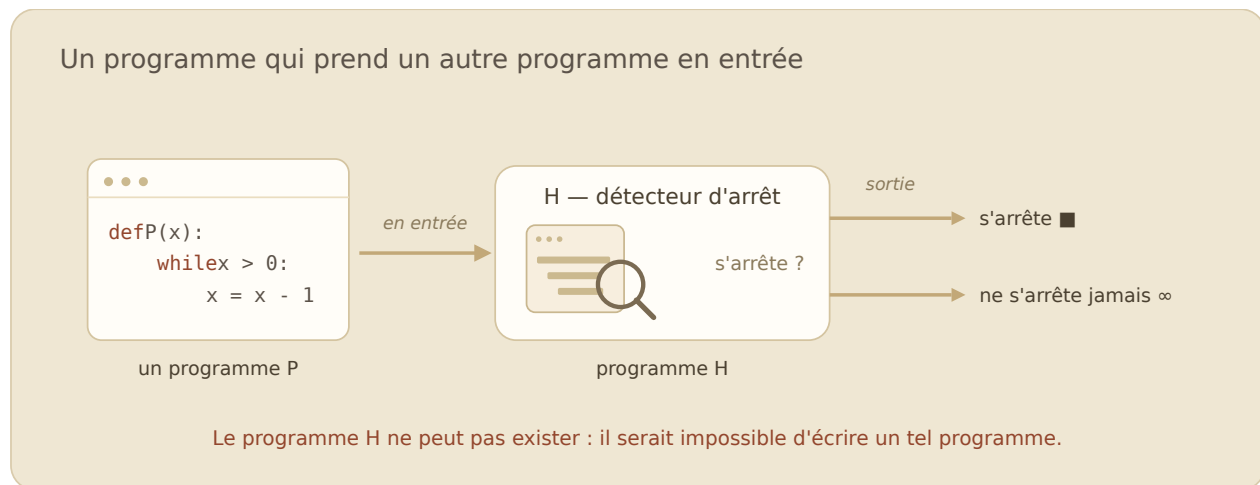
Figure 15: Le problème de l'arrêt (halting problem) : un programme qui prendrait un autre programme en entrée pour prédire s'il s'arrête, et pourquoi il ne peut pas exister.
