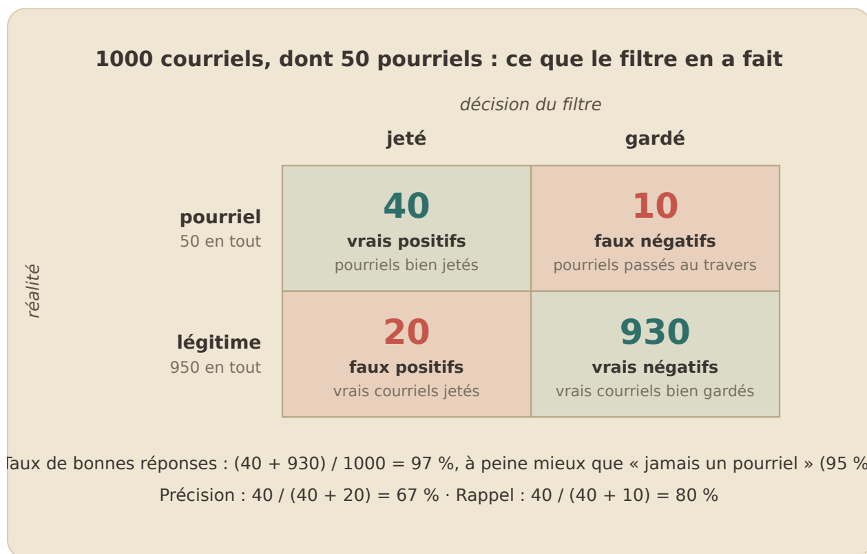
Figure 80: La matrice de confusion : quatre cases au lieu d'un seul score. Les deux cases rouges sont les deux types d'erreur, qui n'ont pas le même coût.
