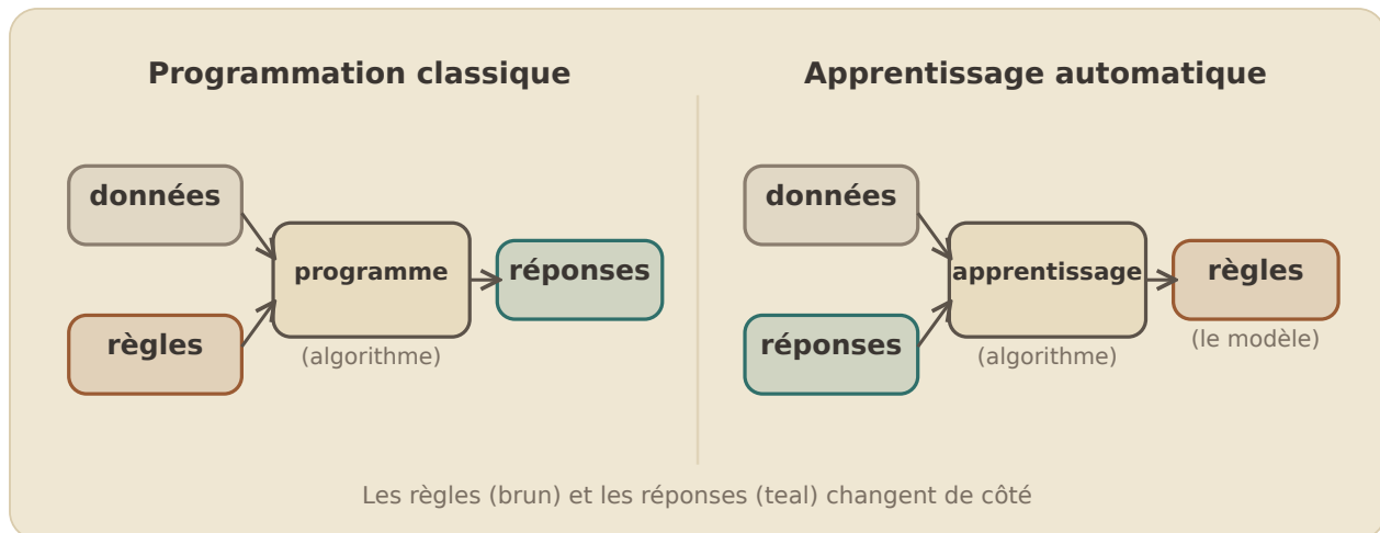
Figure 36: L'inversion au centre de l'apprentissage automatique : ce qu'on fournit et ce que l'ordinateur produit s'inversent. En programmation classique, on écrit les règles ; en AA, c'est l'ordinateur qui les découvre.
