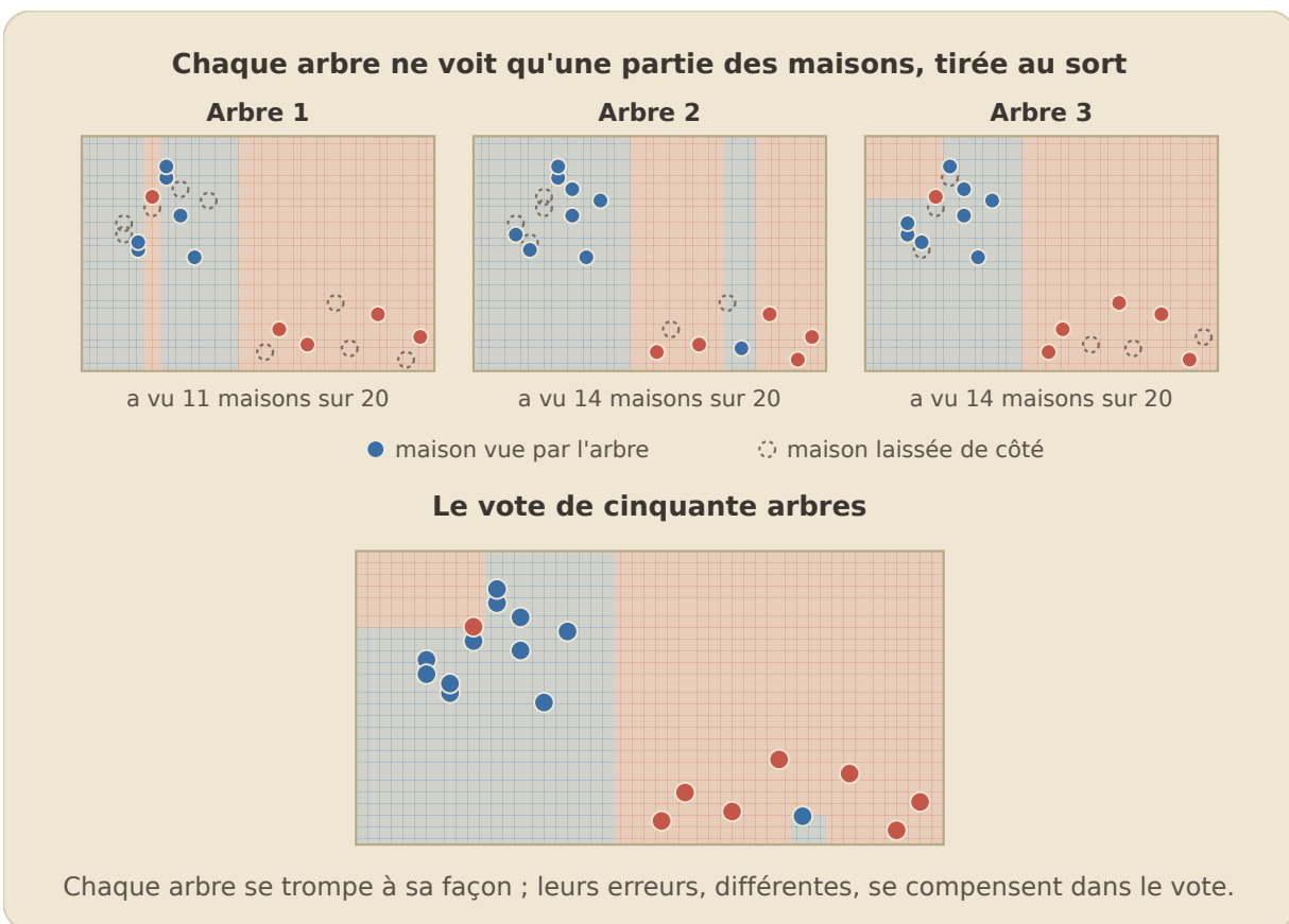
Figure 72: La forêt aléatoire : chaque arbre ne voit qu'une partie des maisons et se trompe différemment ; le vote de cinquante arbres garde ce sur quoi ils s'accordent.
