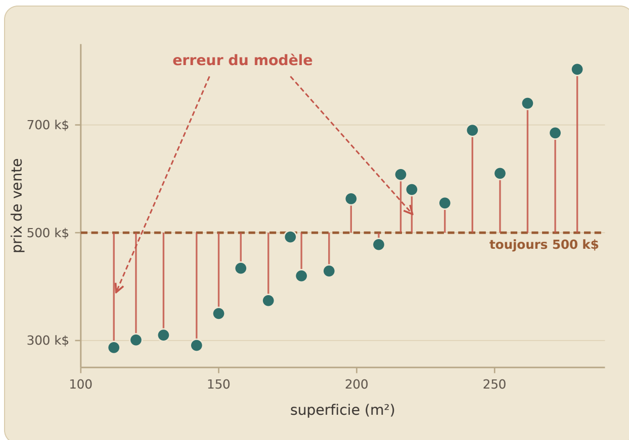
Figure 45: L'erreur du modèle, maison par maison : l'écart vertical entre le vrai prix et la prédiction.
