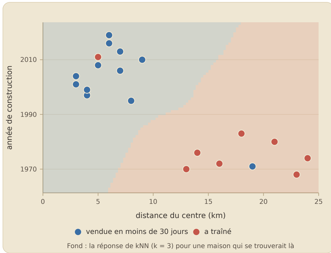
Figure 58: La frontière de décision de kNN ( k = 3 ) sur nos maisons : le fond donne la réponse du modèle en chaque point du plan, et la ligne où la couleur change est la frontière.
