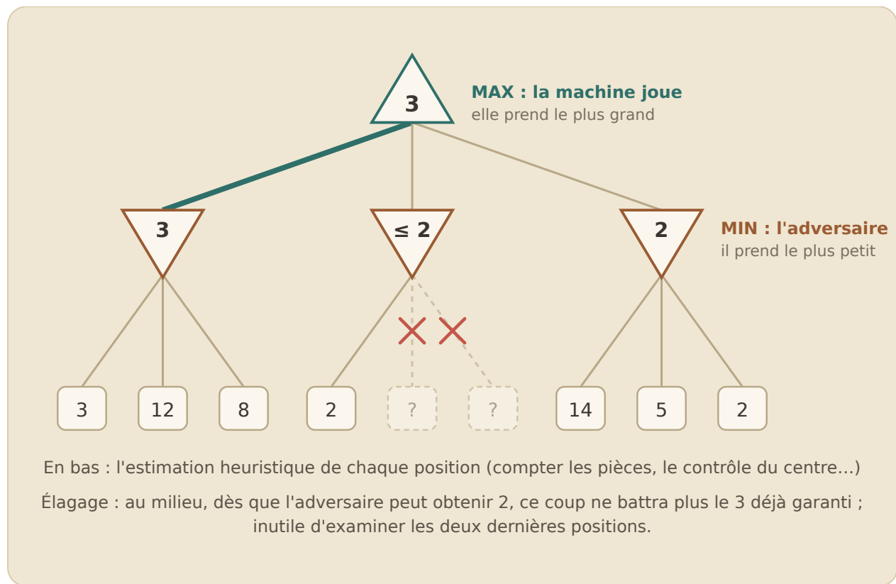
Figure 23: Minimax sur un petit arbre : les estimations remontent, en alternant le plus petit (l'adversaire) et le plus grand (la machine) ; au milieu, l'élagage évite d'examiner deux positions inutiles.
