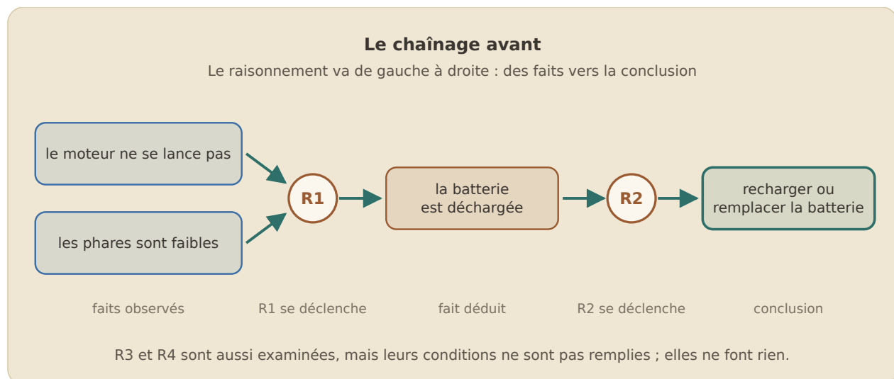
Figure 31: Le chaînage avant : des faits observés vers la conclusion, règle après règle.
