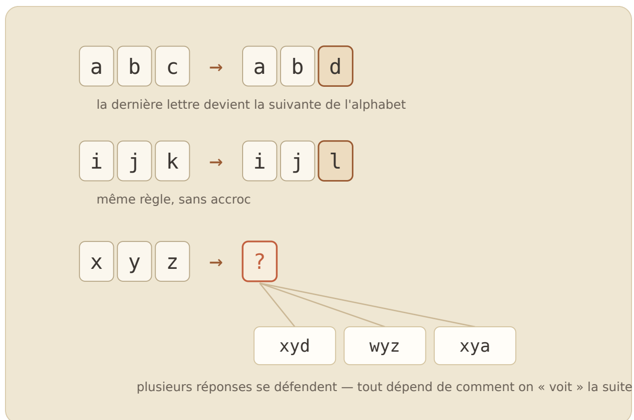
Figure 30: L'énigme de Copycat : pour «xyz», la réponse dépend de la façon dont on perçoit la suite.
