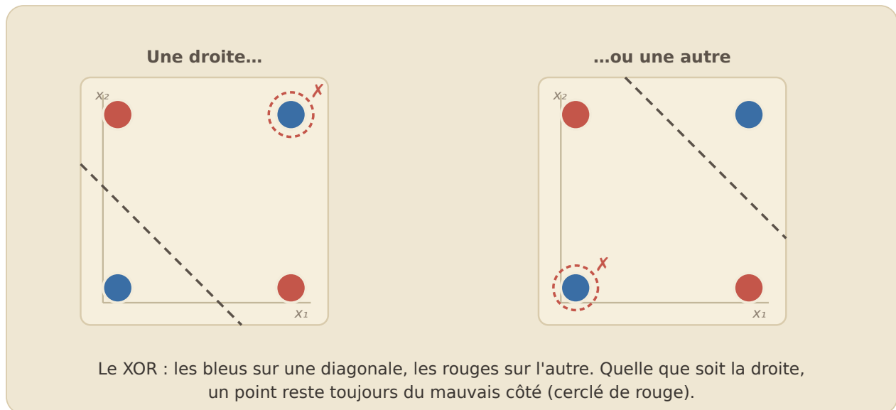
Figure 74: Le XOR : quelle que soit la droite tracée, un point reste du mauvais côté. C'est la limite d'un modèle linéaire.
