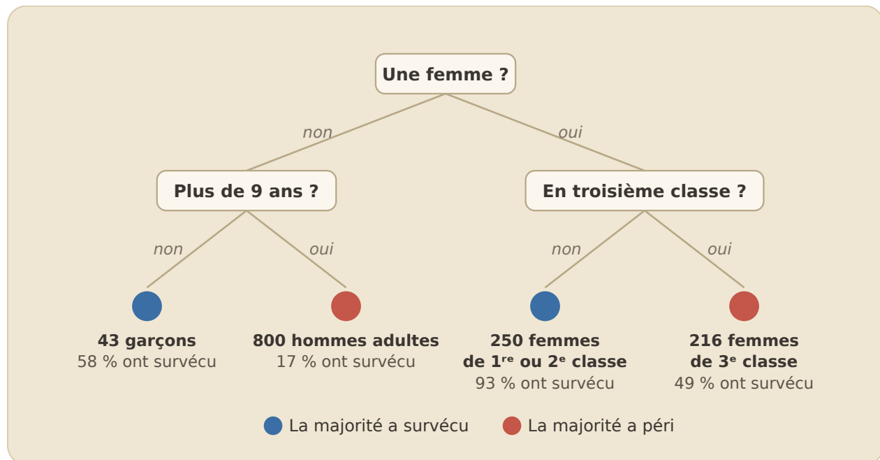
Figure 71: L'arbre du Titanic , appris sur les vraies données : trois questions, 79 % de bonnes réponses, et une histoire qu'on peut lire.
