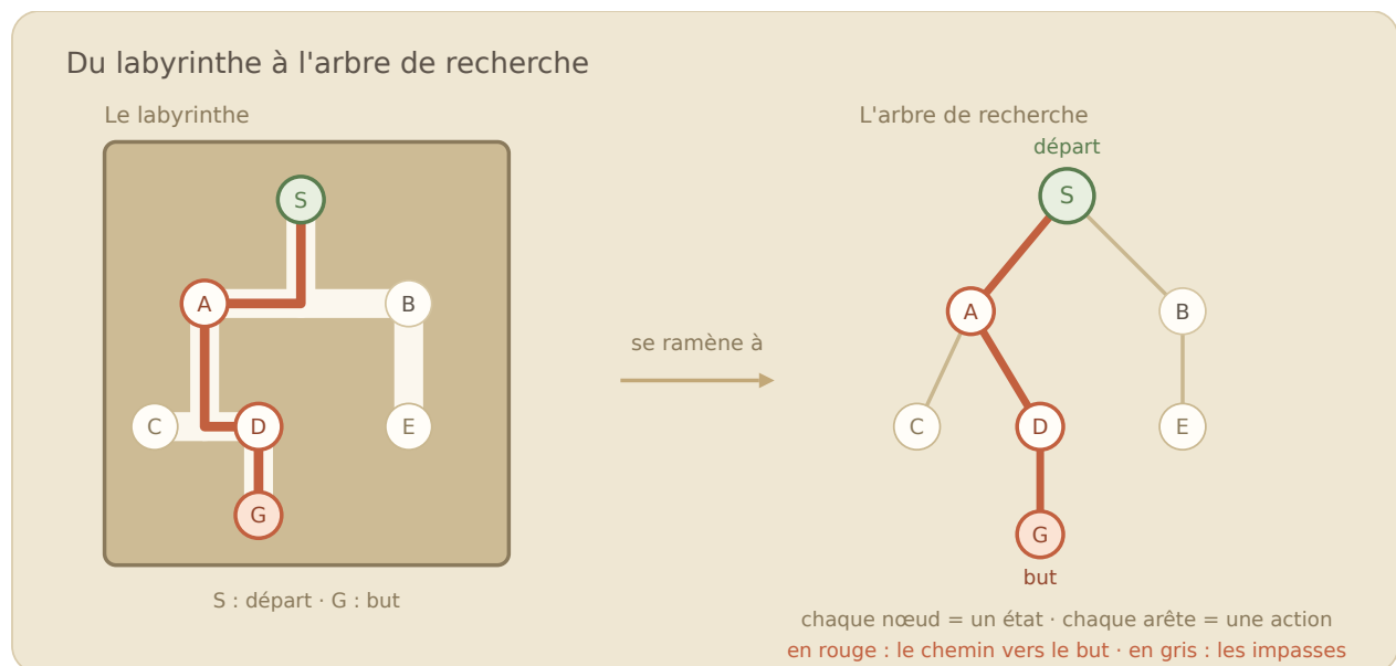
Figure 21: Un labyrinthe est un arbre d'états : résoudre, c'est trouver un chemin de S (départ) à G (but).
