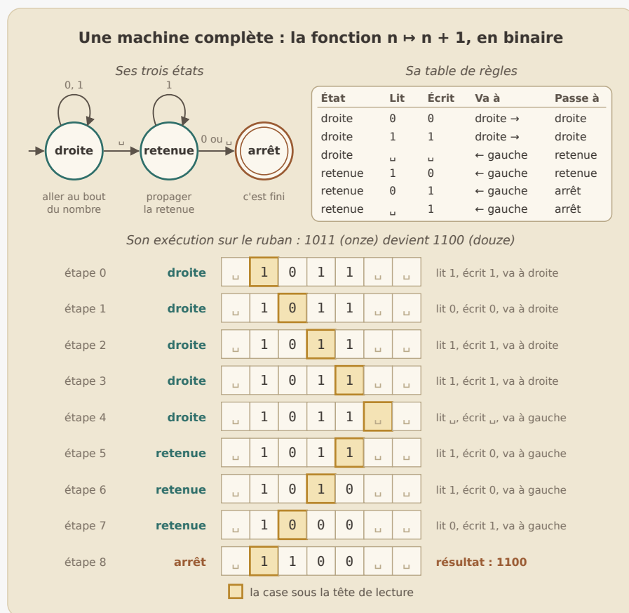
Figure 13: Une machine de Turing complète : trois états, six règles, et la fonction n \mapsto n + 1 exécutée pas à pas sur le ruban.
