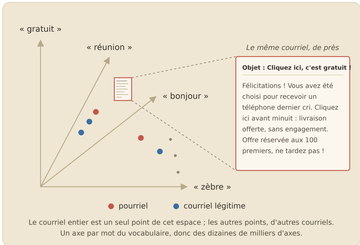
Figure 54: Un axe par mot du vocabulaire, des dizaines de milliers d'axes : le courriel entier devient un seul point de cet espace, comme l'image en devenait un dans celui de ses pixels.
