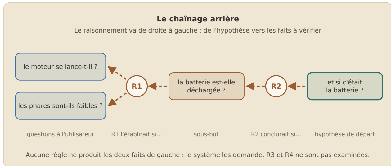
Figure 32: Le chaînage arrière : de l'hypothèse vers les faits à vérifier, en ne posant que les questions utiles.
