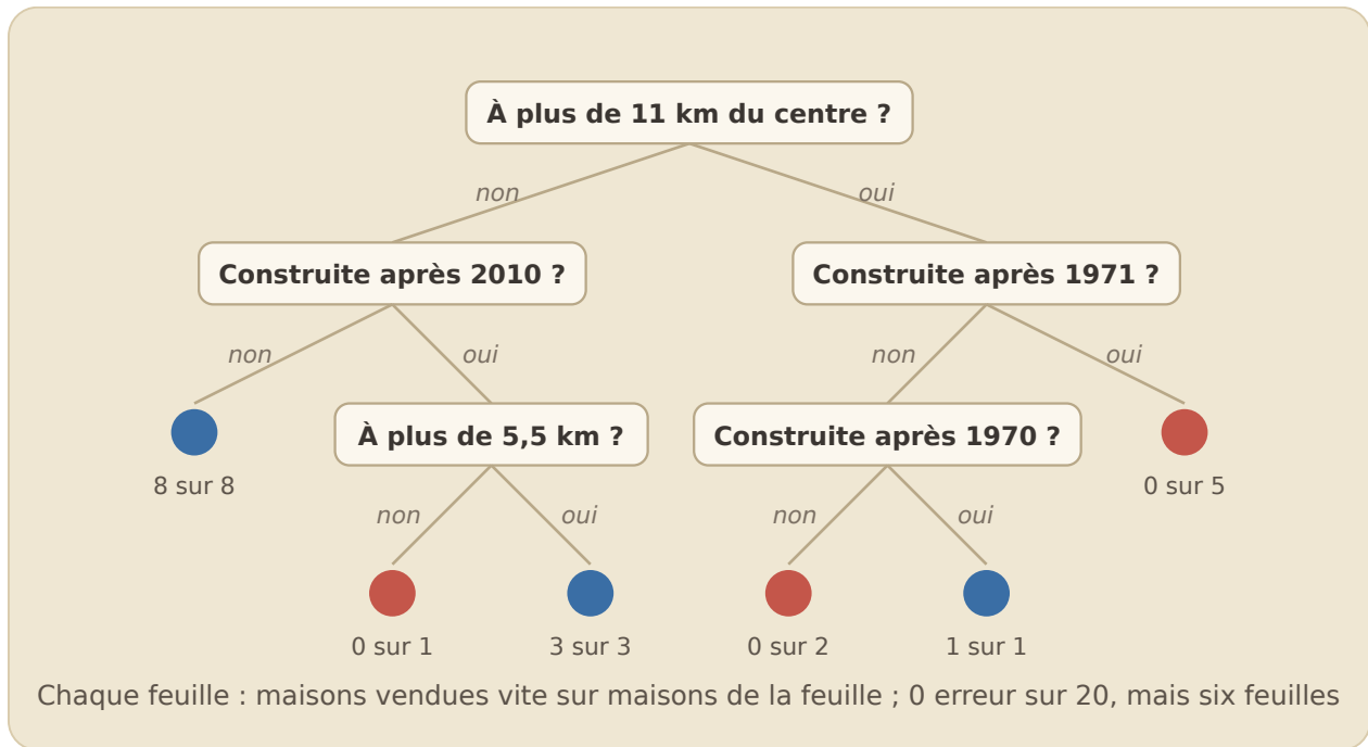
Figure 69: Le même arbre, laissé pousser sur trois niveaux : six feuilles, zéro erreur, et une feuille sur mesure pour chaque exception.
