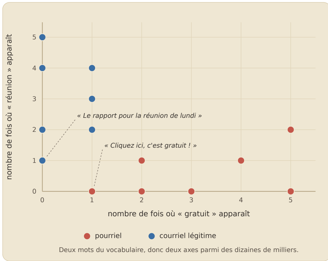
Figure 53: Deux mots du vocabulaire, deux axes : chaque courriel devient un point, et les pourriels se rangent d'un côté, les courriels légitimes de l'autre.
