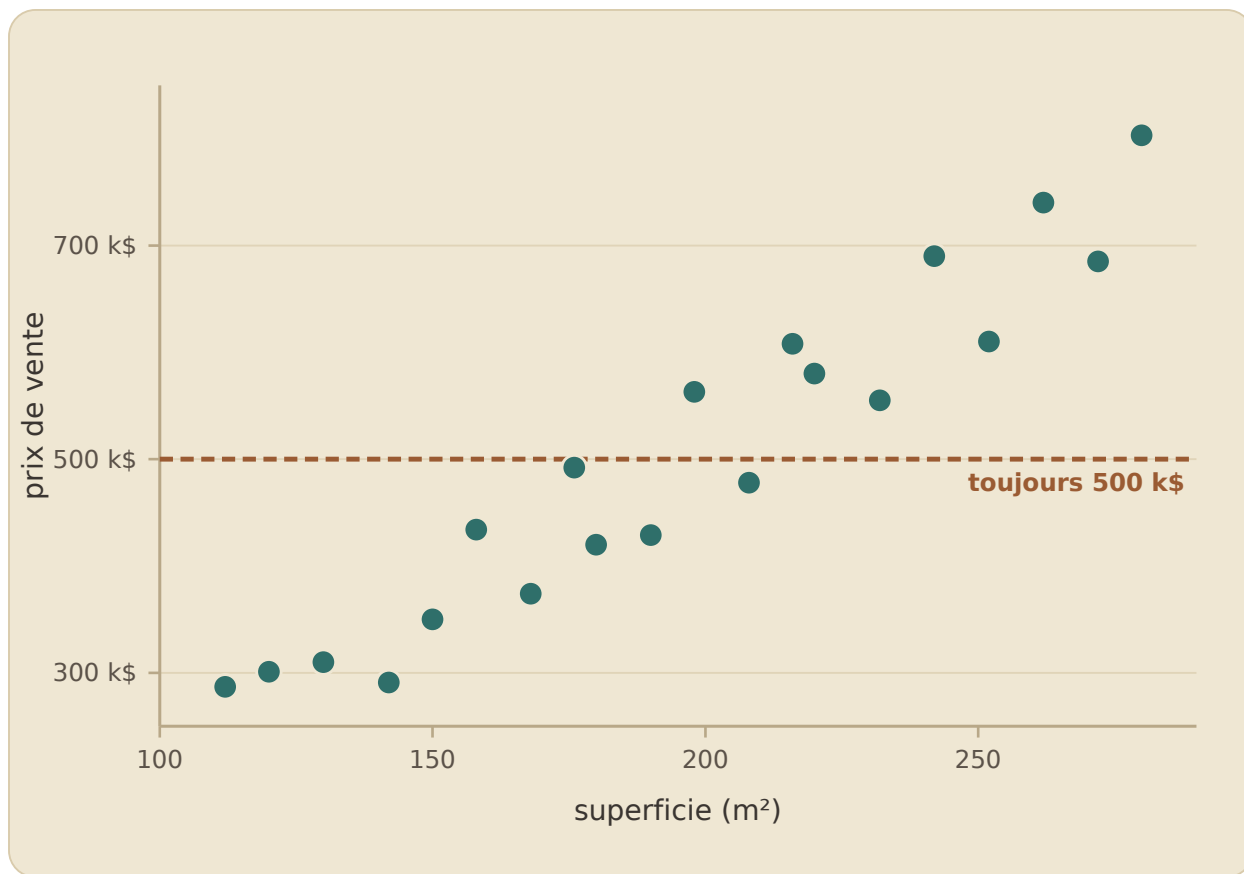
Figure 44: Le modèle le plus bête : une droite plate à 500 000 $, qui ignore complètement la superficie.
