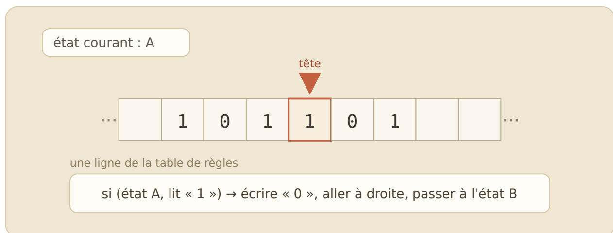
Figure 12: Une machine de Turing : lire un symbole, l'écrire, se déplacer, changer d'état.
