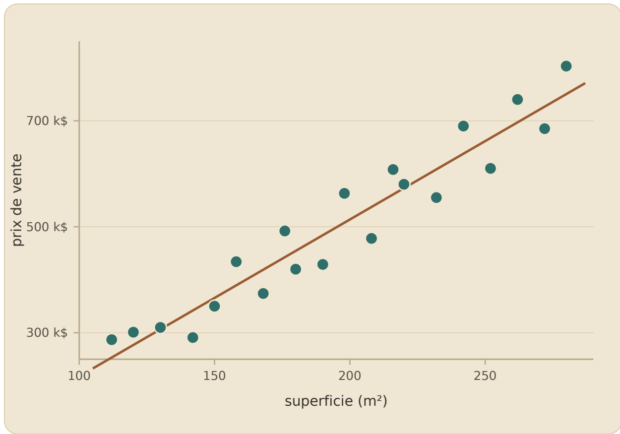
Figure 60: La droite qui suit la tendance du nuage : c'est notre modèle.
