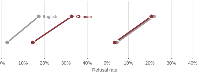
deepseek-chat-v3.1
