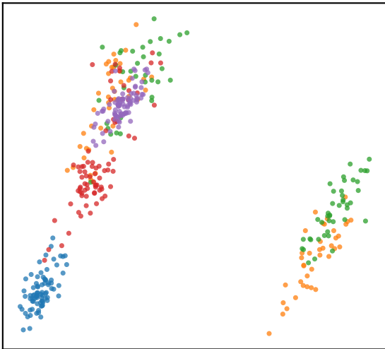
Pretrained – PCA
