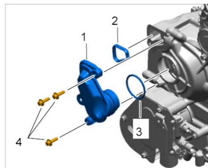
曲轴箱强制通风装置的盖 1-3
