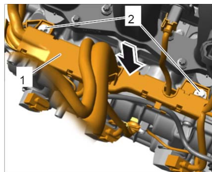
固定喷油器的电缆扎带
