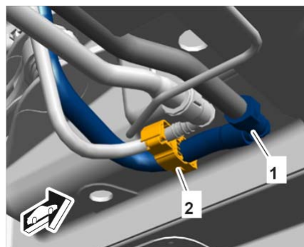
管路托架
