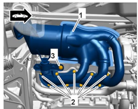
排气歧管螺钉视图, 1-3 侧
