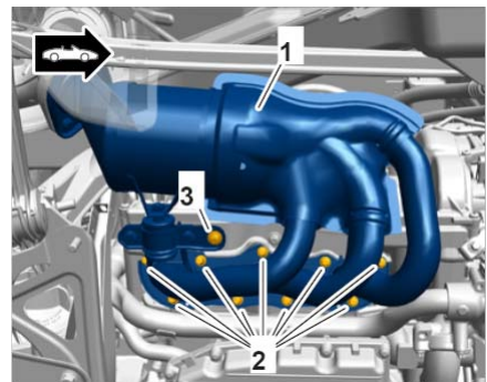
排气歧管螺纹接头视图，1-3 列
