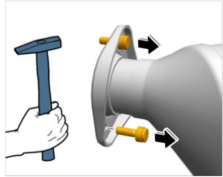
敲出排气歧管上的螺栓
