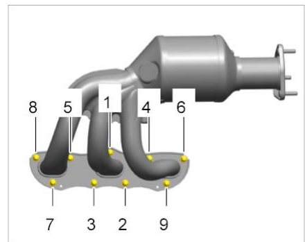
排气歧管的紧固顺序
