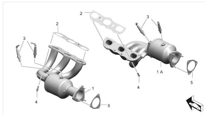
排气歧管的部件概图（以 991 车型为例）
