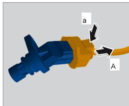
脉冲传感器上的接头
