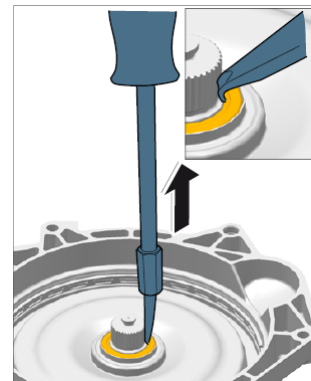
拆卸密封环
