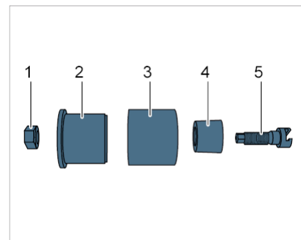
Porsche Doppelkupplung (PDK) 保时捷双离合器变速箱密封环的装配工具
