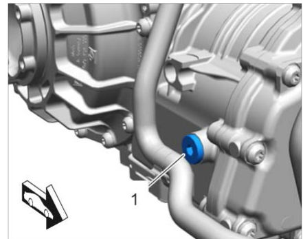
机油加注口螺钉/检油塞
