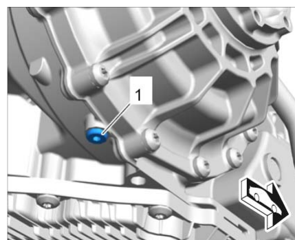
差速器空间的放油塞
