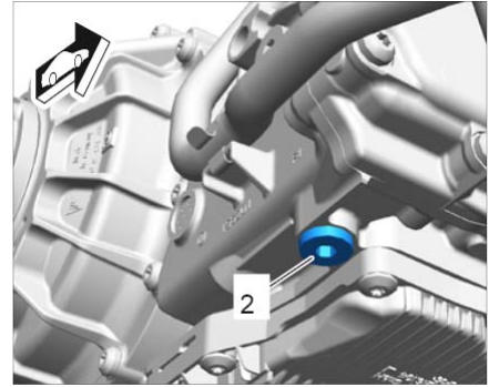
齿轮组空间的放油塞
