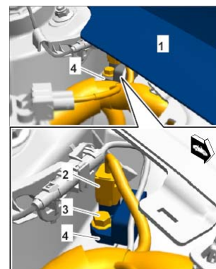
松开车身前传感器
