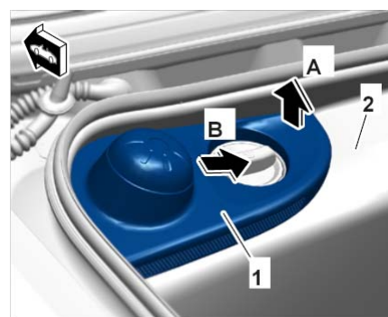
松开弹簧滑柱盖
