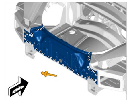
安装后封闭板
