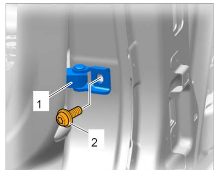
拆卸车身侧车门限位器
