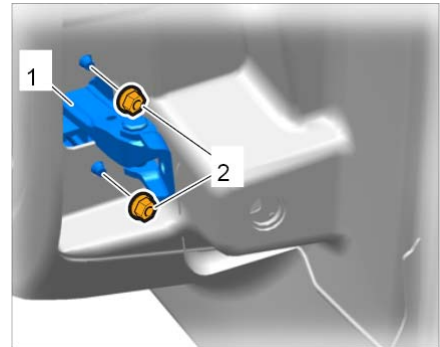
拆卸车门限位器
