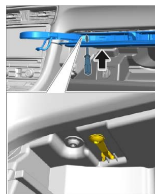
松开杯座
