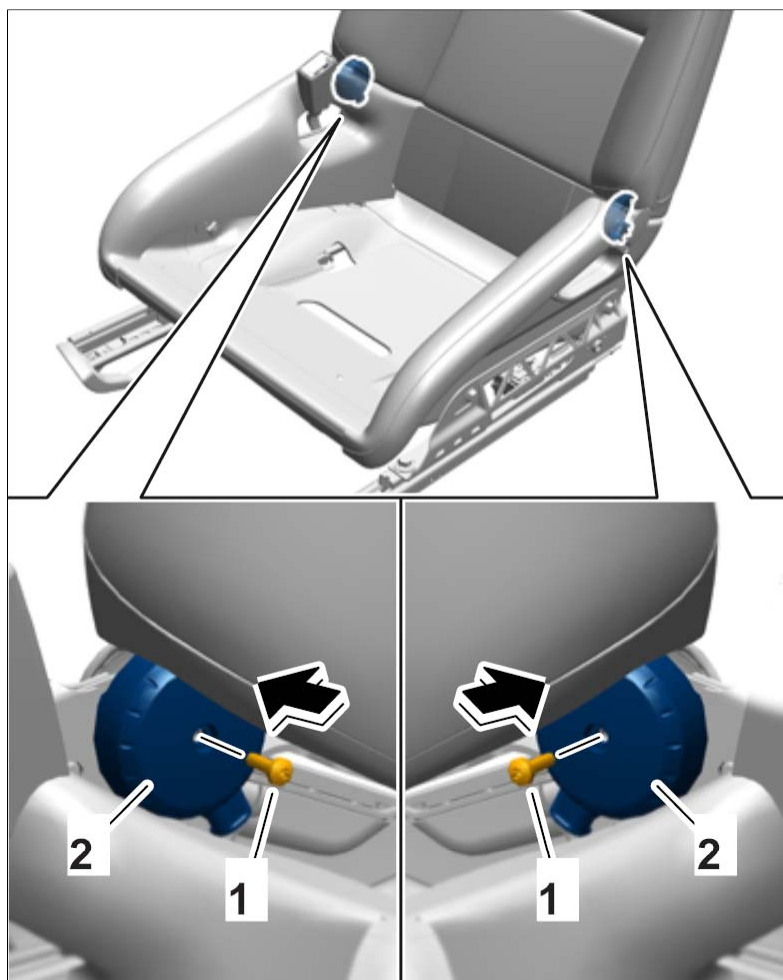
安装内侧铰链的饰件
