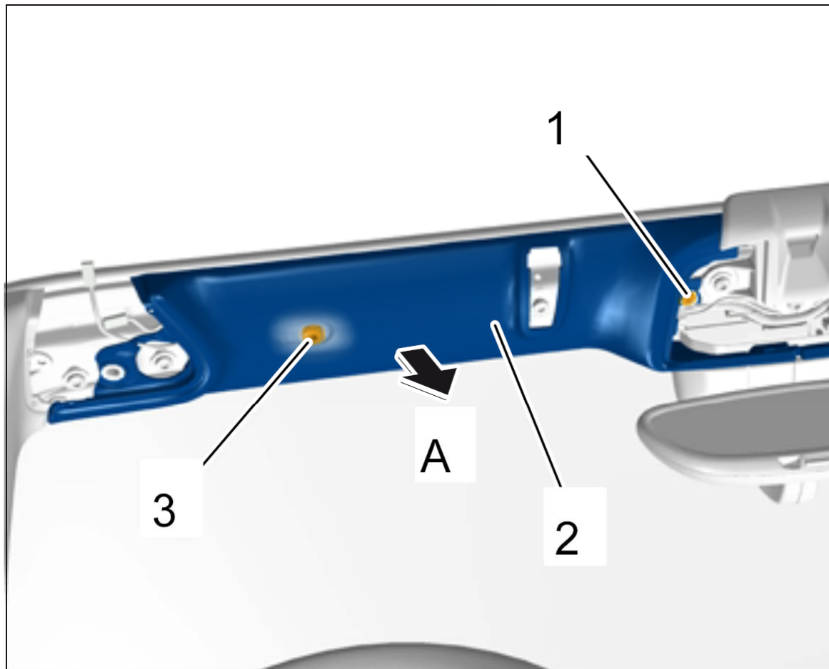
拆卸侧面的前车顶饰板
