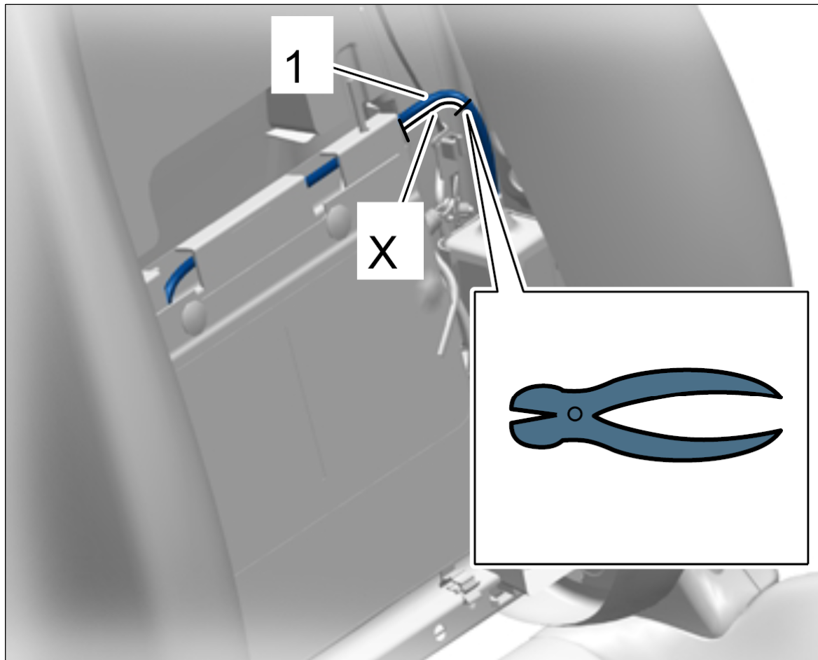
切断空气连接管路
