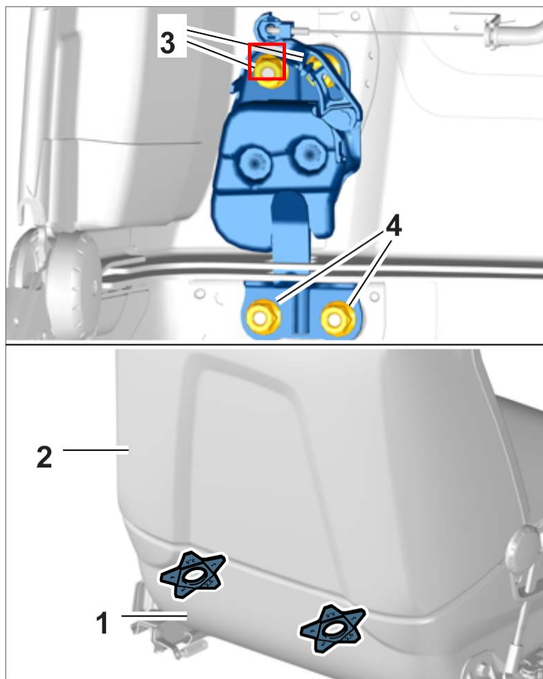
调节靠背调节装置的锁
