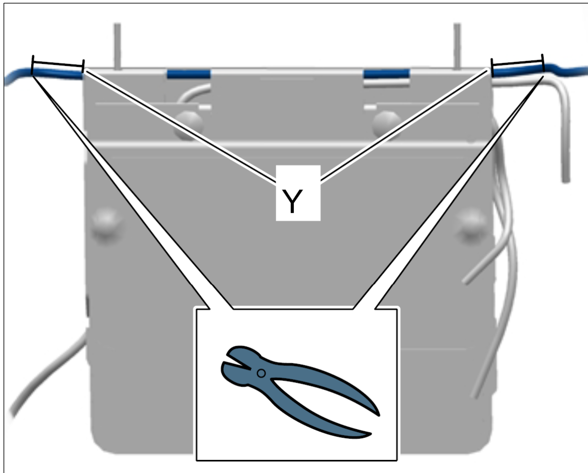
气垫空气连接管路
