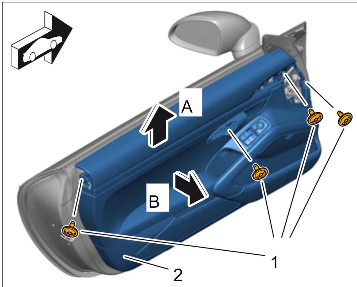
门板支座
