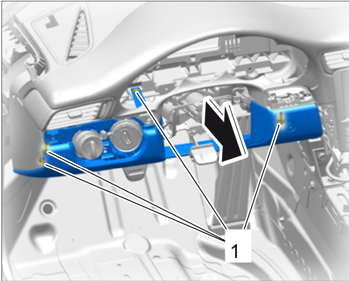
松开饰板
