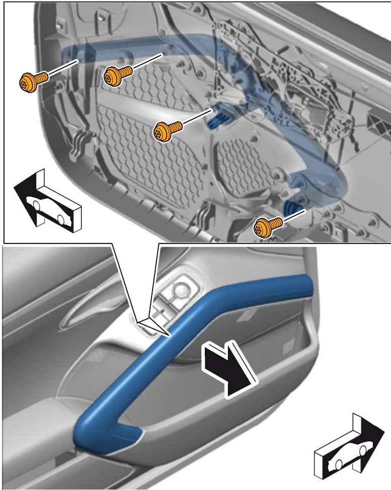
拆卸把手
