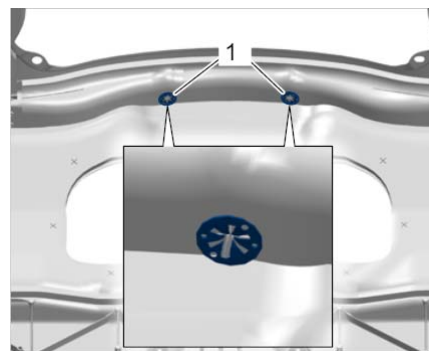
拆卸固定卡子
