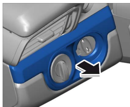
拆卸驾驶员侧（左侧）的仪表板模塑件
