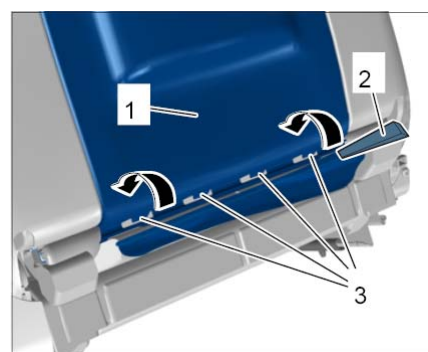
固定座椅罩
