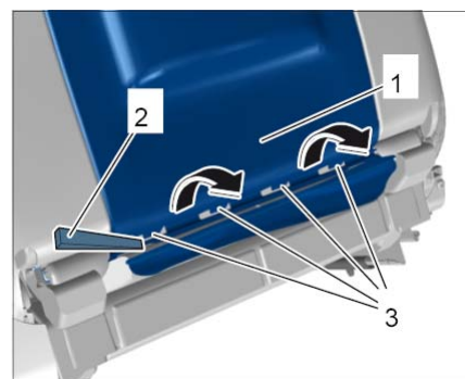
松开后罩
