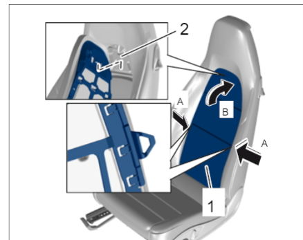
固定前部的罩
