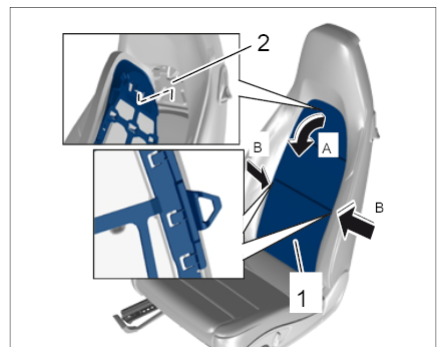
松开前部的罩
