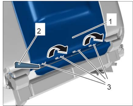
松开后罩
