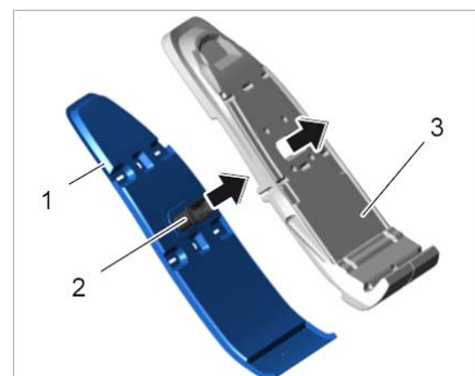
安装前排中间靠背的加热元件
