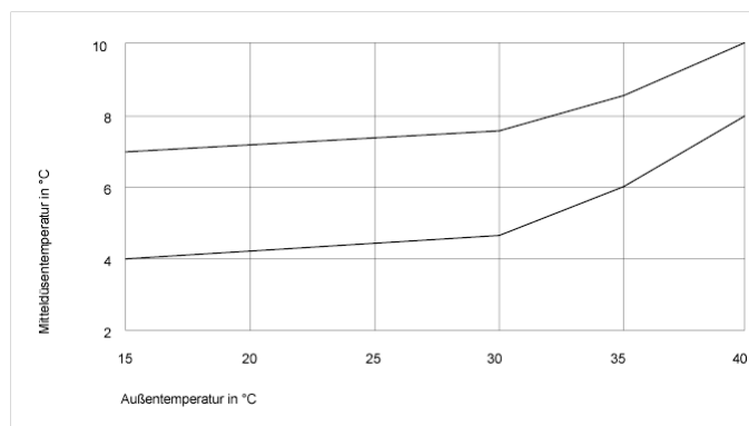
中央通风口温度是环境温度的函数
