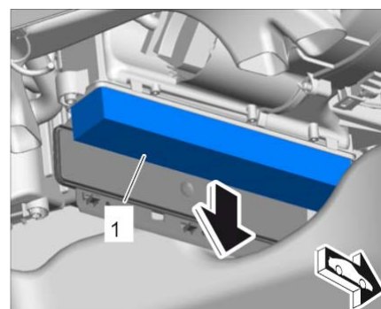
拔出微粒过滤器
