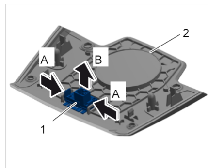
拆卸日照传感器
