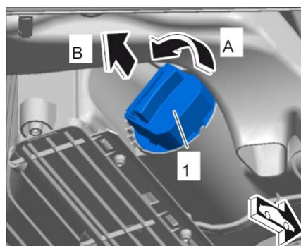
拆卸风扇控制按钮
