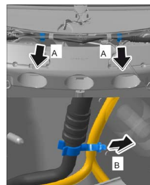
松开管路支座
