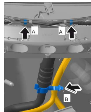
固定管路
