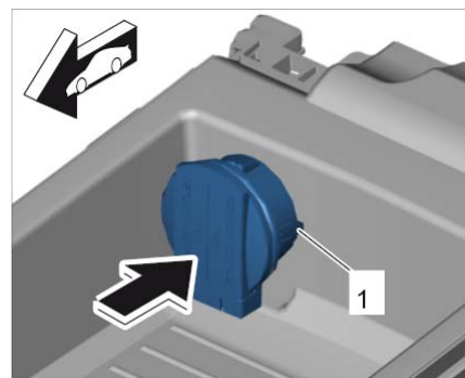
安装带罩的紧固环
