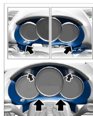
固定仪表板插件
