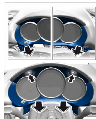
拆卸仪表板插件
